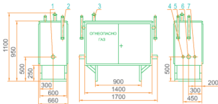
габаритная схема ГРПШ-400-01
