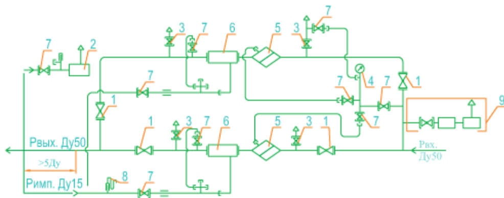
функциональная схема ГРПШ-03БМ-2У1
