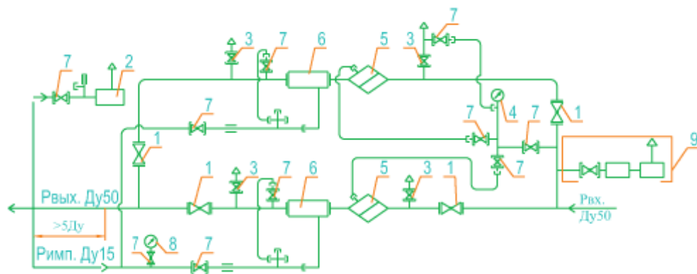
функциональная схема ГРПБ-03М1-2У1
