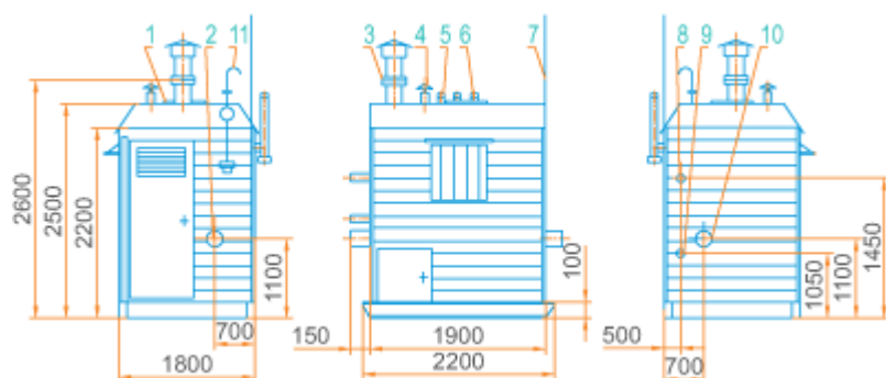
габаритная схема ГРПБ-03М1-2У1
